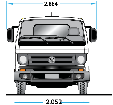
Dimensiones principales (mm)
