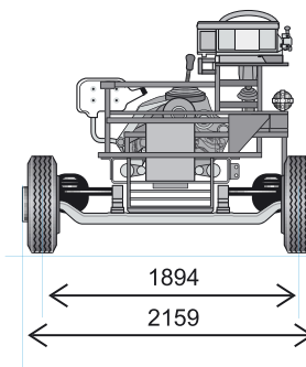
Dimensiones principales (mm)
